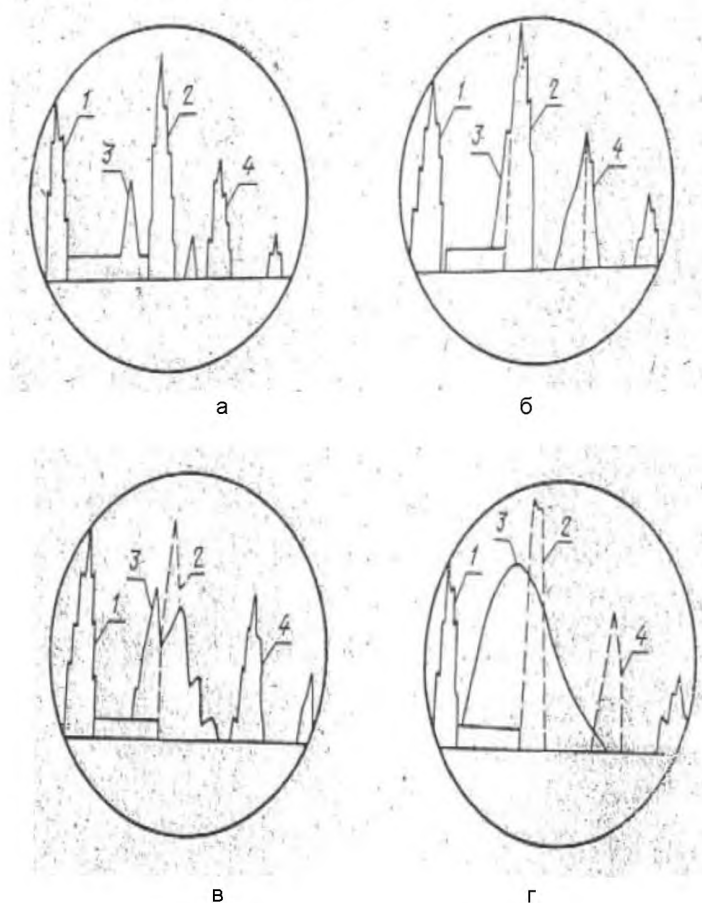
Рисунок В.1— Вид эхо-сигналов на экране дефектоскопа
